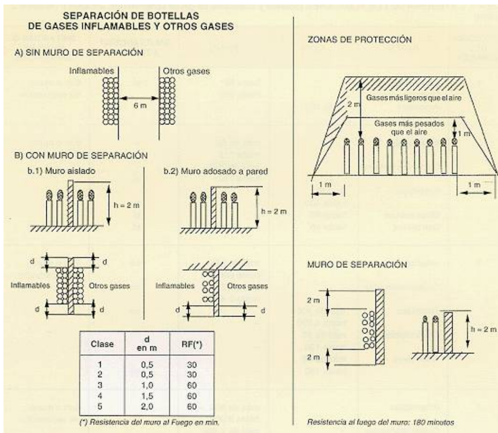
Fig. 1: Almacenamiento de gases licuados en recipientes móviles
