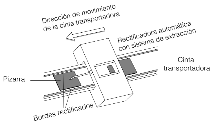
Figura 1. Rectificadora de pizarra automática
