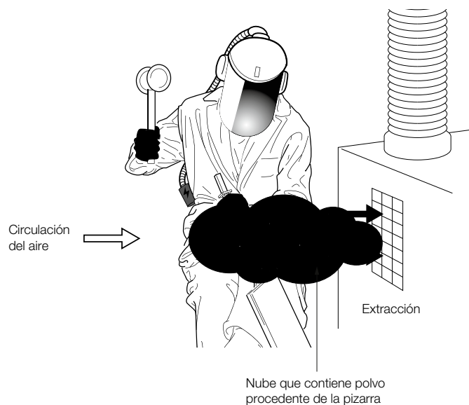
Figura 1. Labrado manual de pizarra utilizando extracción localizada
